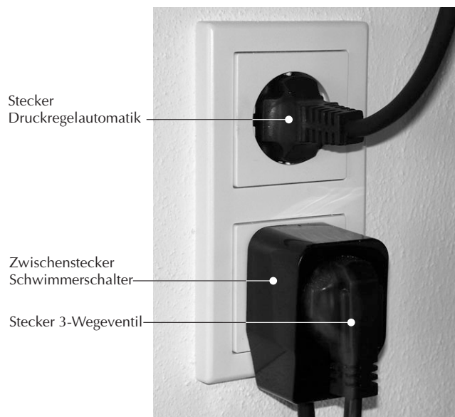
Bild 8 Elektrischer Anschluss der Box 10
