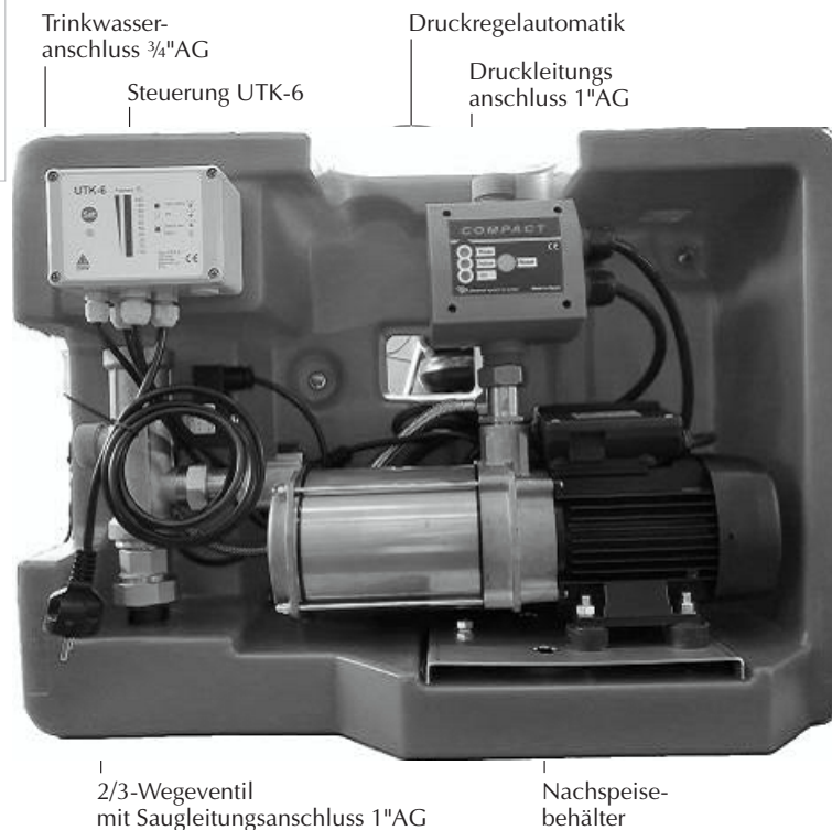
Bild 4 Aufbau
