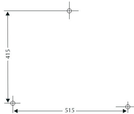
Bild 7 Lochschablone für Wandmontage Box V20
