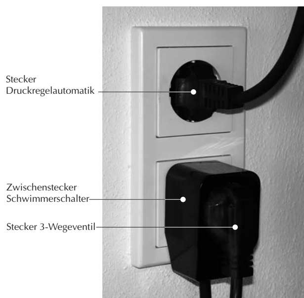
Bild 8 Elektrischer Anschluss der Box V20
