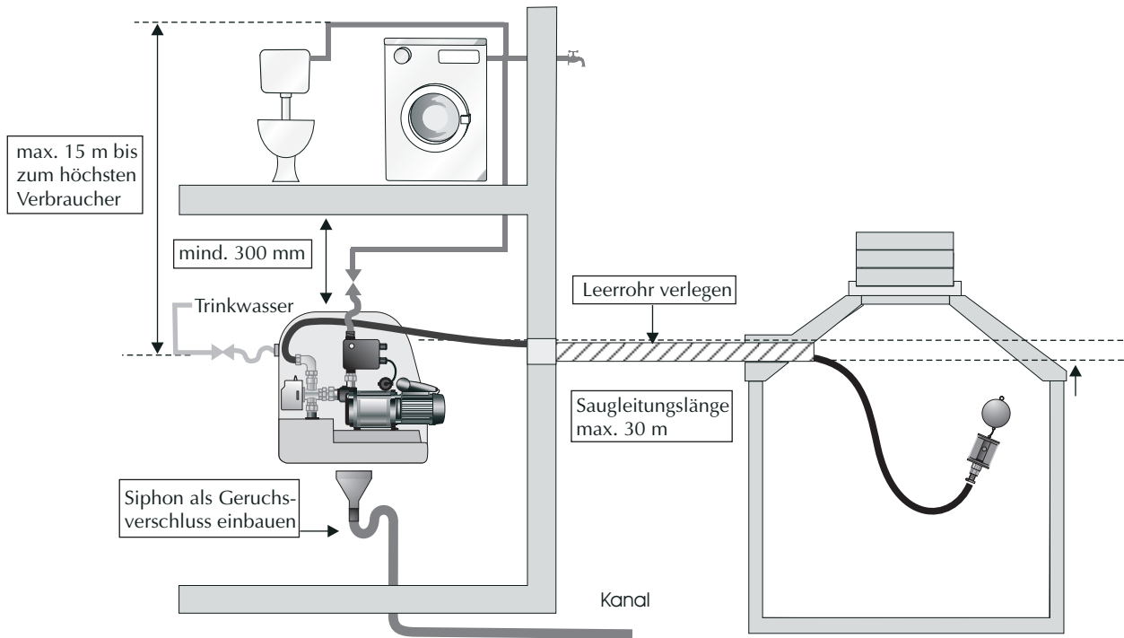
Bild 9 Hydraulischer Anschluss der Box V20
