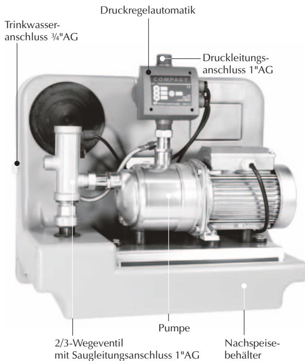
Bild 4 Aufbau
